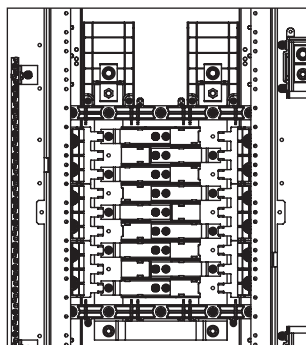
Monophasé
