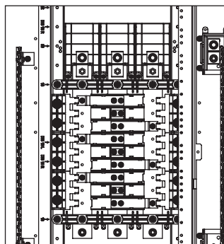
Triphasé
